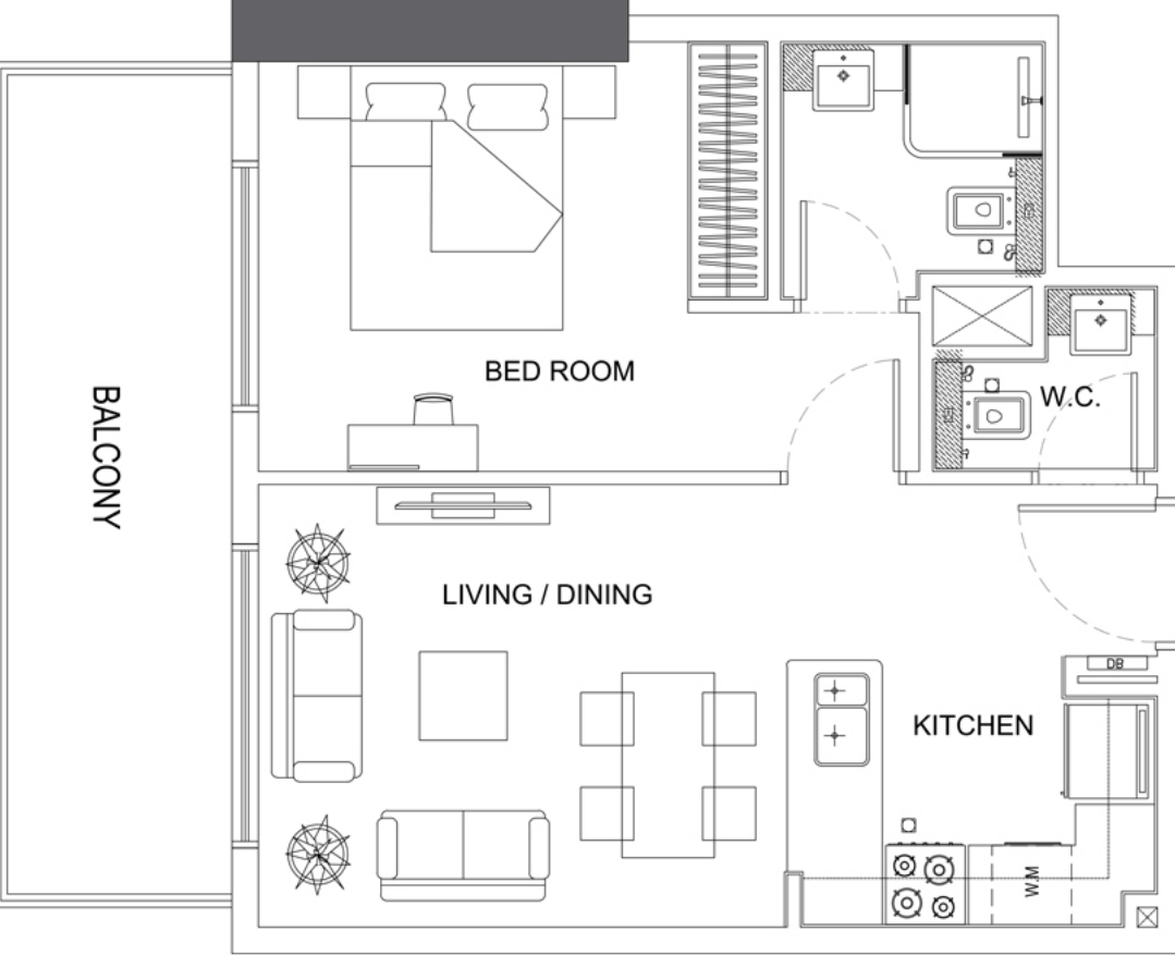
1 BEDROOM TYPE 01
