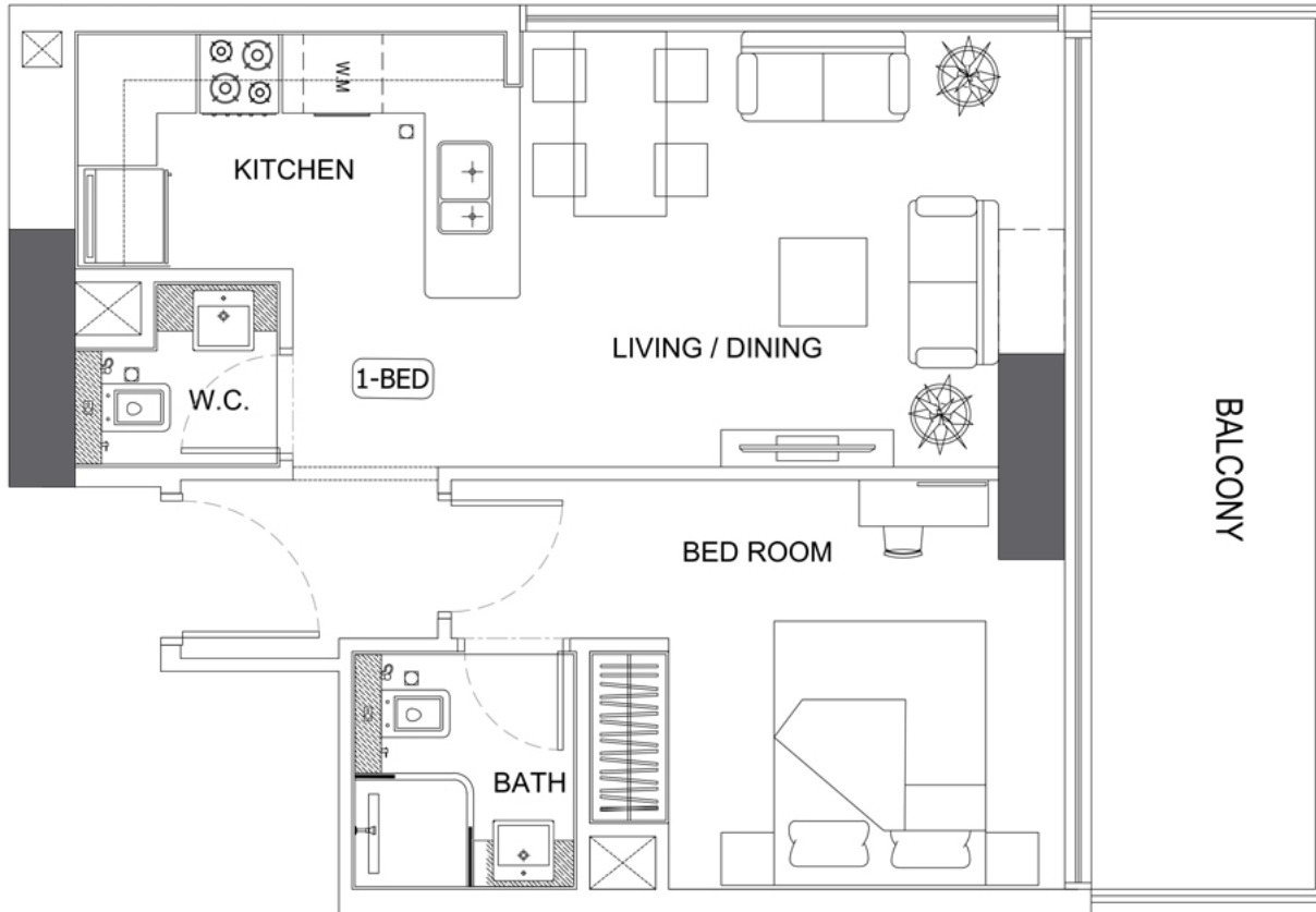
1 BEDROOM TYPE 05
