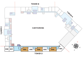
LEVEL-01 (PODIUM 01)
