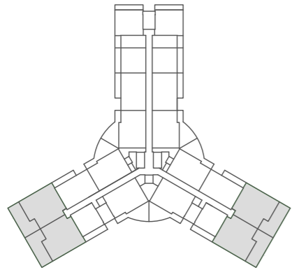
Floor : 06
