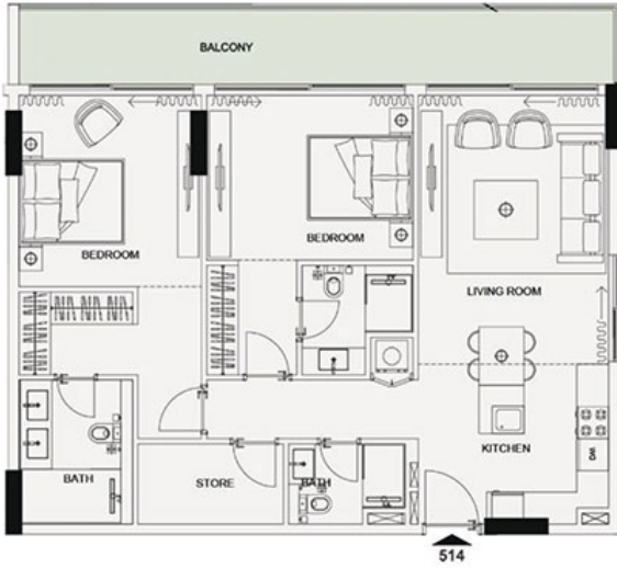
UNIT 514 - 2 BEDROOM
