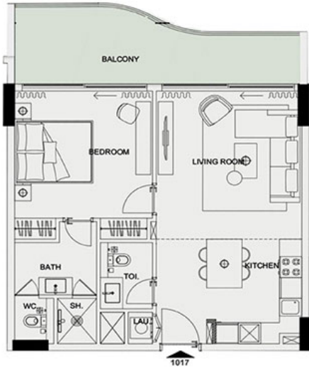
UNIT 1017 - 1 BEDROOM
