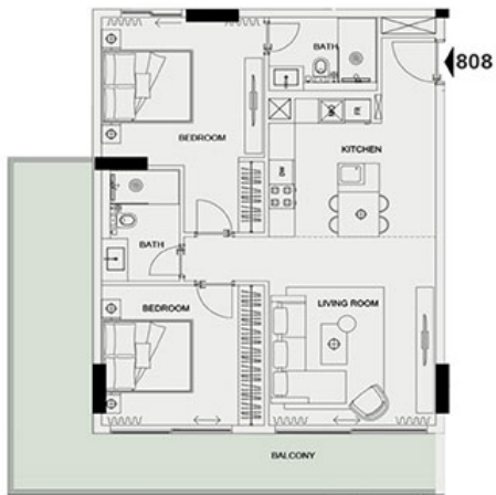
UNIT 808 - 2 BEDROOM
