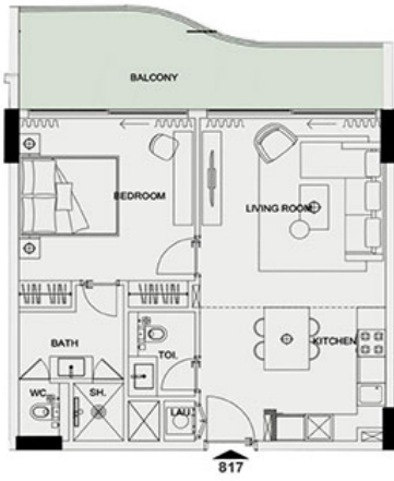
UNIT 817 - 1 BEDROOM
