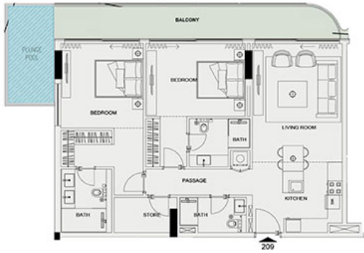
UNIT 209 - 2 BEDROOM
