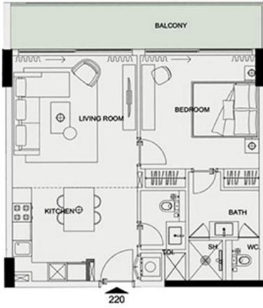
UNIT 220 - 1 BEDROOM
