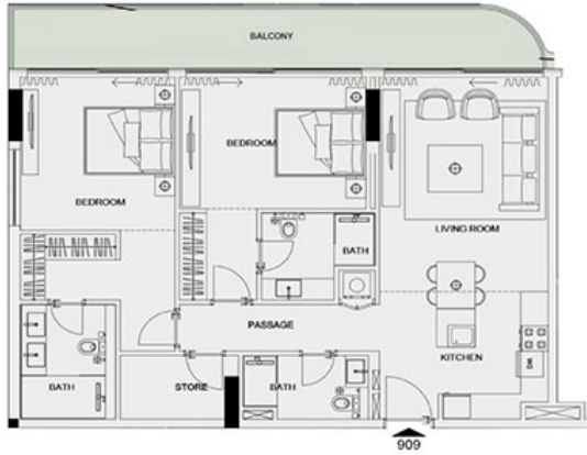
UNIT 909 - 2 BEDROOM
