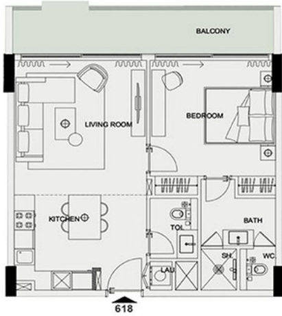
UNIT 618 - 1 BEDROOM
