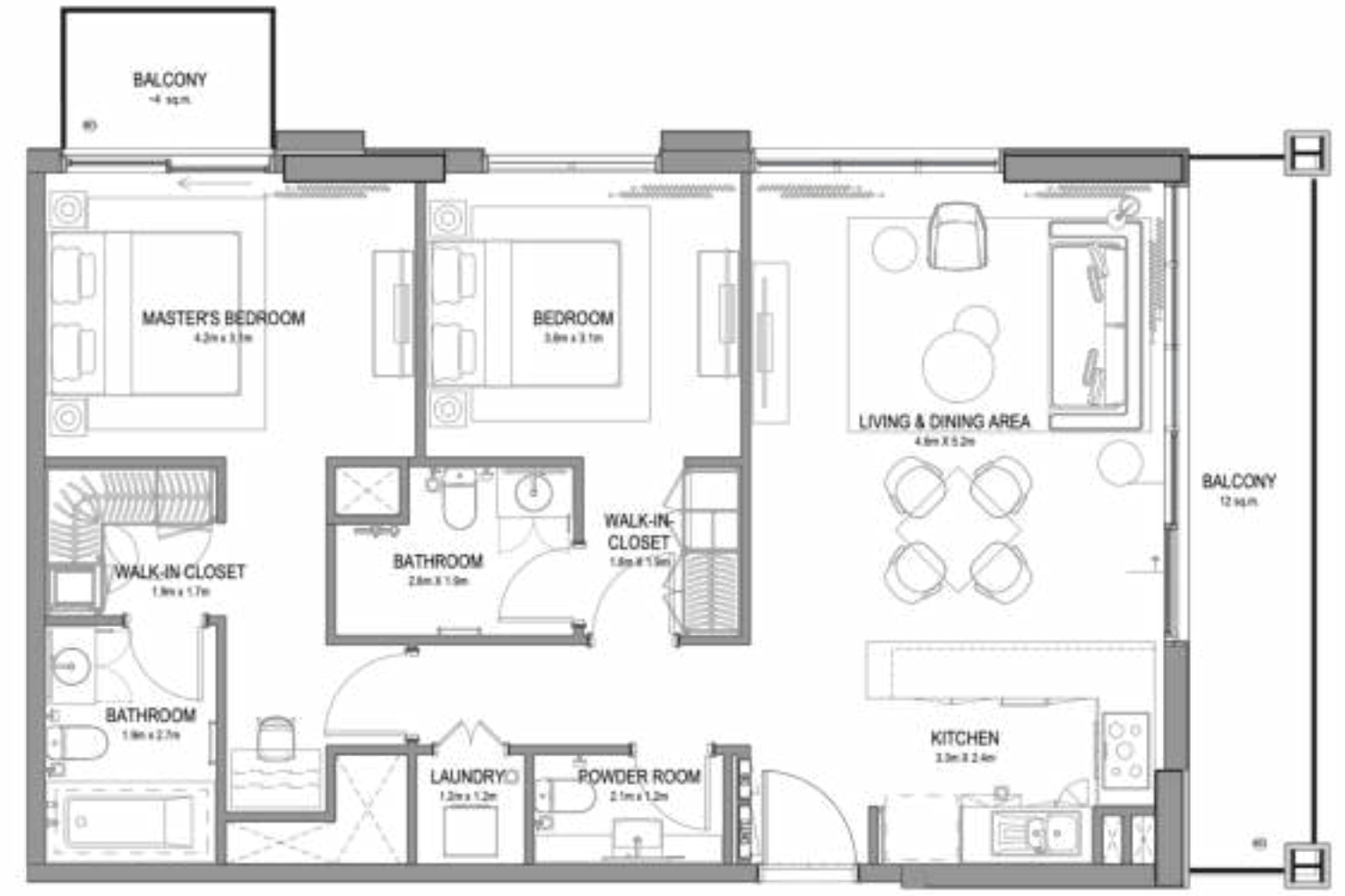
2 BEDROOMS TYPE - 4
